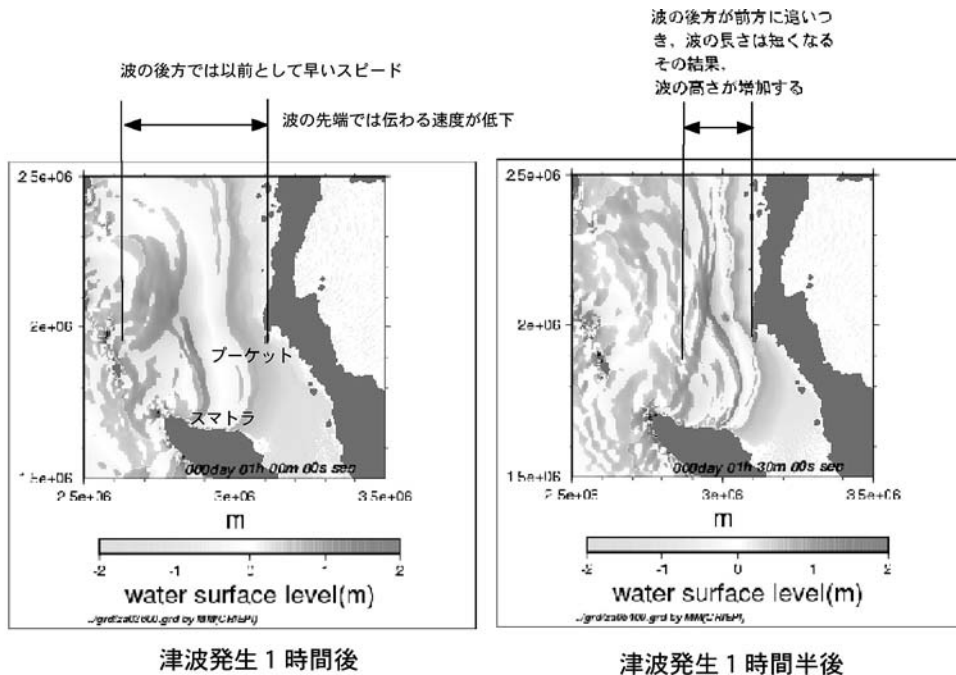
図一 3 波源から東側へ伝わる津波 (波長が急激に短くなり、その分波高が増幅する、電中研・松山氏解析結果に加筆)
