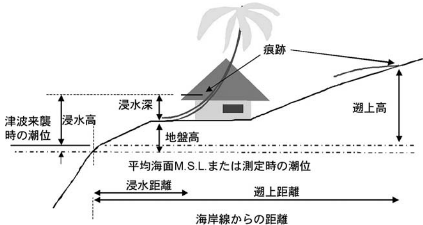
図-4 津波高さ・深さの定義
