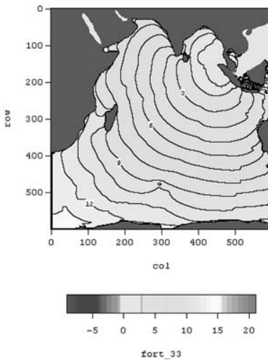
図一 2 津波伝播図
