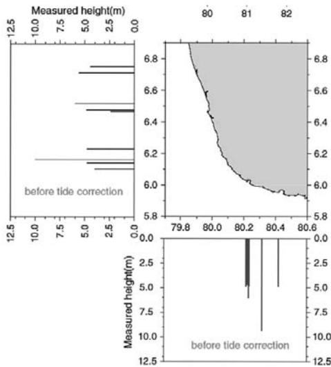
図一 5 (b) 合同調査団による津波浸水高・遡上高
