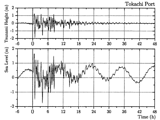
(a) 十勝港で観測された潮位（下段）とFFTを利用して抽出した津波成分（上段、地震発生6時間前～48時間後、1分間隔記録）
