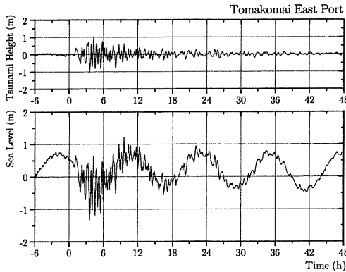
図-13 苫小牧東港で観測された潮位（下段）とFFTを利用して抽出した津波成分（上段）（地震発生6時間前～48時間後，1分間隔記録）
