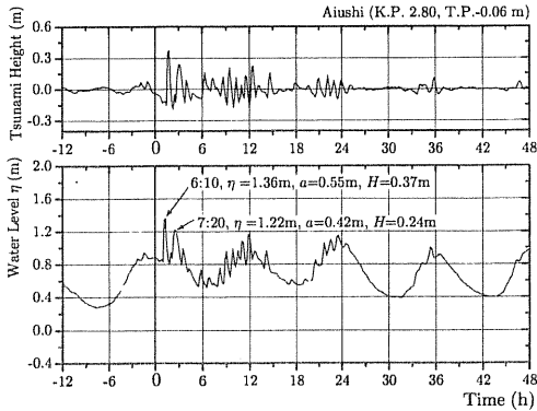
図-6 愛牛水位観測所の10分間隔水位記録（下段）とFFTを実施して抽出した津波成分（上段、地震発生12時間前～48時間後）
