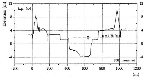
図-4 十勝川本川k.p.5.4の横断面と大津水位観測所の最大水位の関係
