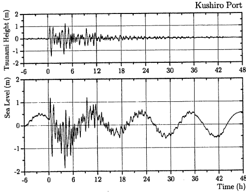
(a) 釧路港で観測された潮位（下段）とFFTを利用して抽出した津波成分（上段）（地震発生6時間前～48時間後，1分間隔記録6）。ただし，速報値。）
